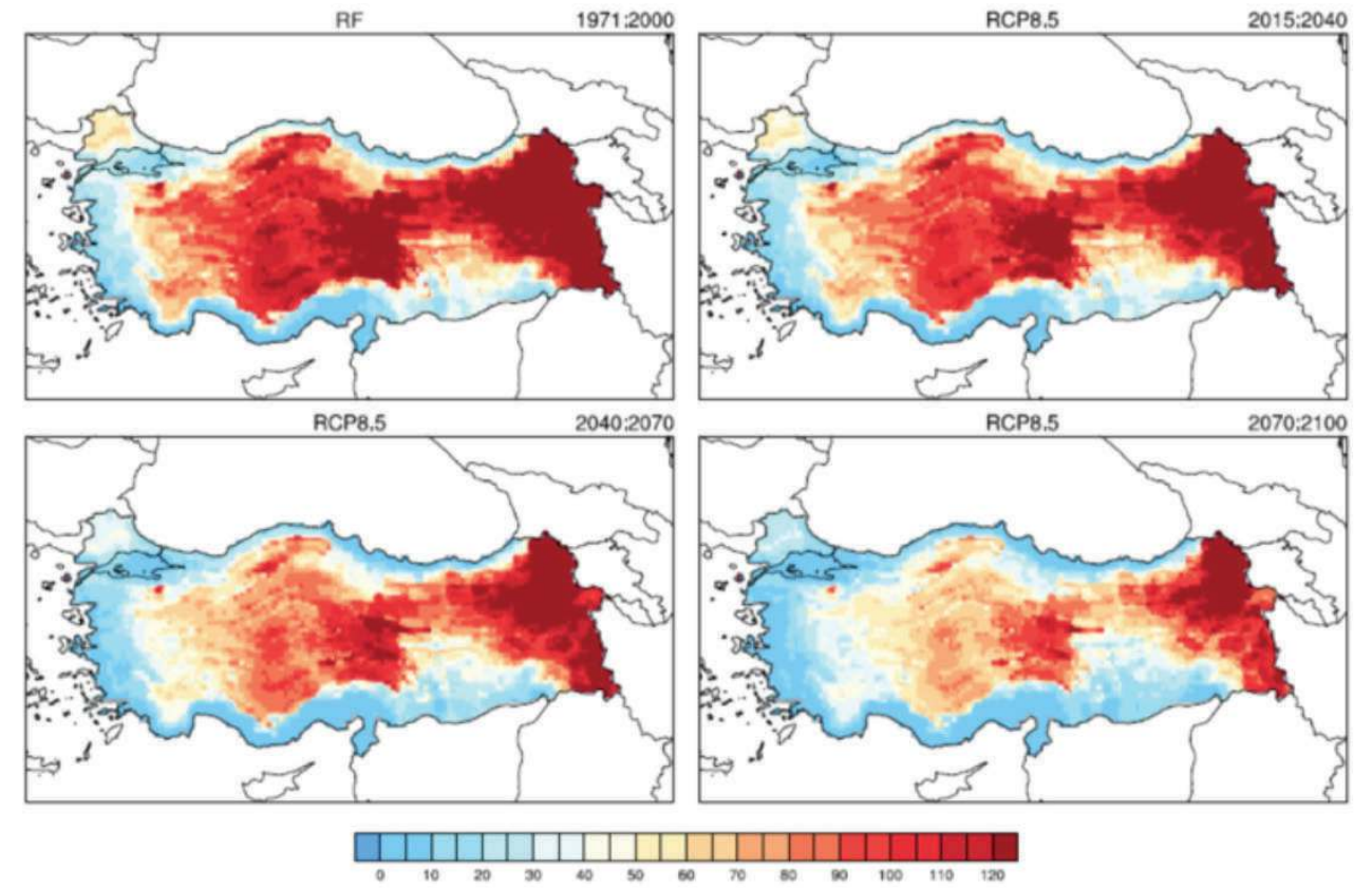
Şekil 3.2.7. MPI-ESM-MR Modeli RCP8.5 Senaryosuna göre 30 yıllık Donlu Günler (FDO) İklim İndisi değerlerinin belirtilen periyot içerisindeki yıllık ortalamaları (gün) (SYGM, 2016).
