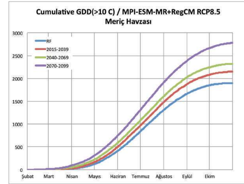
Şekil III.17. Havza ortalaması alınmış Meriç Tarım Havzası için RCP8.5 senaryosuna göre hesaplanmış olan, ortalama günlük toprak sıcaklığı 10°C ve üzeri büyüme derece günlerinin yıl içindeki eklenik toplamalarına ait mevcut durum 1971-2000 (mavi çizgi) ile birlikte bu mevcut duruma göre 2015-39 (kırmızı çizgi), 2040-69 (yeşil çizgi) ve 2070-99 (mor çizgi) dönemleri için küresel iklim değişimi ile oluşan eğilim projeksiyonları.
