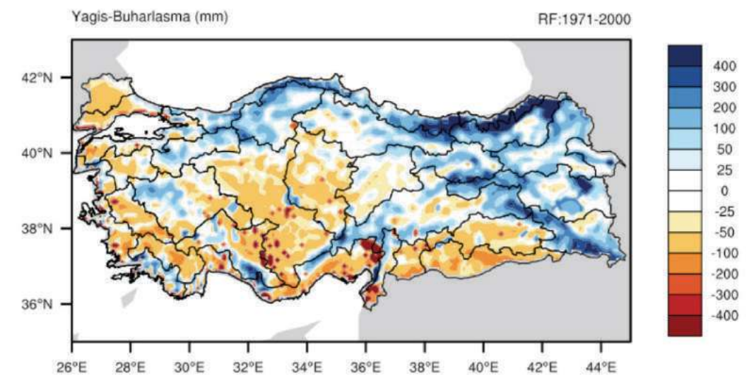
Şekil 3.3.10. MPI-ESM-MR+RegCM Modeli RCP8.5 Senaryosuna göre 1971-2000 referans dönemi bitki büyüme mevsiminde (Mart-Ekim) beklenen yıllık toplam yağış ile gerçek buharlaşma-terlemenin farkları.
