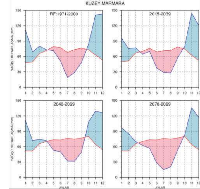
Şekil IV.19. Havza ortalaması alınmış Kuzey Marmara Tarım Havzası için RCP8.5 senaryosuna göre hesaplanmış olan, ortalama aylık toplam yağışın (mavi çizgi) ve gerçekleşen buharlaşma-terlemenin (kırmızı çizgi) yıl içindeki değişimine ait mevcut durum 1971-2000 ile birlikte bu mevcut duruma göre 2015-39, 2040-69 ve 2070-99 dönemleri için küresel iklim değişimi ile oluşan eğilim projeksiyonları.
