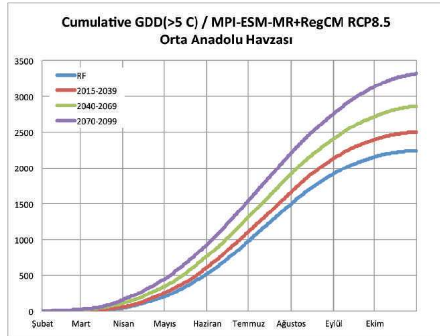
Şekil 3.2.8. Orta Anadolu Tarım Havzası için ortalama günlük toprak sıcaklığı 5°C ve üzeri büyüme derece günlerinin yıl içindeki eklenik toplamına ait mevcut durum 1971-2000 (mavi çizgi) ile birlikte RCP8.5 senaryosuna göre gelecek 2015-39 (kırmızı çizgi), 2040-2069 (yeşil çizgi) ve 2070-2099 (mor çizgi) dönemleri için küresel iklim değişimi ile oluşan eğilim projeksiyonları.
