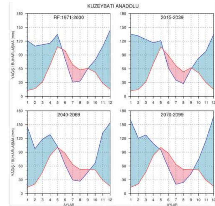
Şekil IV.20. Havza ortalaması alınmış Kuzeybatı Anadolu Tarım Havzası için RCP8.5 senaryosuna göre hesaplanmış olan, ortalama aylık toplam yağışın (mavi çizgi) ve gerçekleşen buharlaşma-terlemenin (kırmızı çizgi) yıl içindeki değişimine ait mevcut durum 1971-2000 ile birlikte bu mevcut duruma göre 2015-39, 2040-69 ve 2070-99 dönemleri için küresel iklim değişimi ile oluşan eğilim projeksiyonları.
