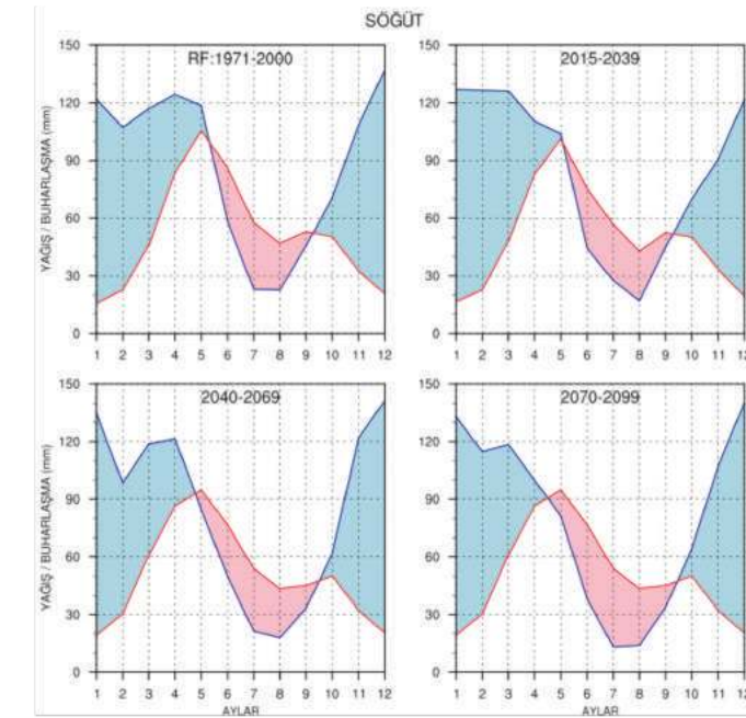
Şekil IV.24. Havza ortalaması alınmış Söğüt Tarım Havzası için RCP8.5 senaryosuna göre hesaplanmış olan, ortalama aylık toplam yağışın (mavi çizgi) ve gerçekleşen buharlaşma-terlemenin (kırmızı çizgi) yıl içindeki değişimine ait mevcut durum 1971-2000 ile birlikte bu mevcut duruma göre 2015-39, 2040-69 ve 2070-99 dönemleri için küresel iklim değişimi ile oluşan eğilim projeksiyonları.
