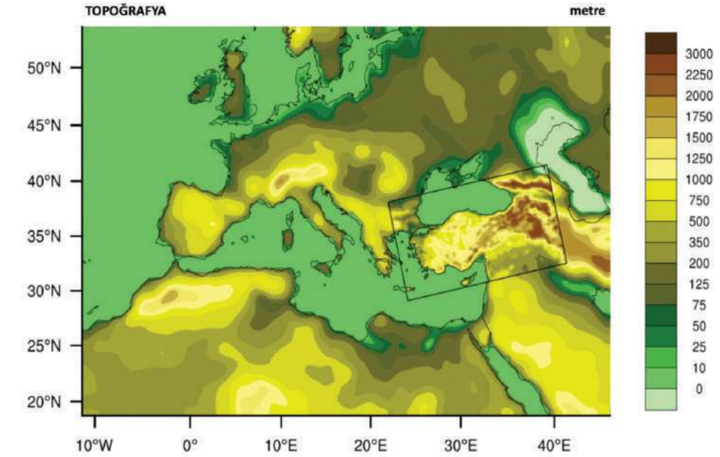
Şekil 2.1.2. Dıştaki hesap alanı 50 km çözünürlüğe ve içteki alan 10 km çözünürlüğe karşılık gelmek üzere Bölgesel Model Çalışma Alanları ve Topografya (SYGM 2016).
