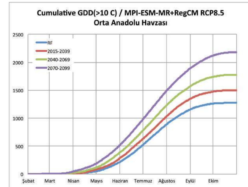
Şekil III.30. Havza ortalaması alınmış Orta Anadolu Tarım Havzası için RCP8.5 senaryosuna göre hesaplanmış olan, ortalama günlük toprak sıcaklığı 10°C ve üzeri büyüme derece günlerinin yıl içindeki eklenik toplamına ait mevcut durum 1971-2000 (mavi çizgi) ile birlikte bu mevcut duruma göre 2015-39 (kırmızı çizgi), 2040-69 (yeşil çizgi) ve 2070-99 (mor çizgi) dönemleri için küresel iklim değişimi ile oluşan eğilim projeksiyonları.
