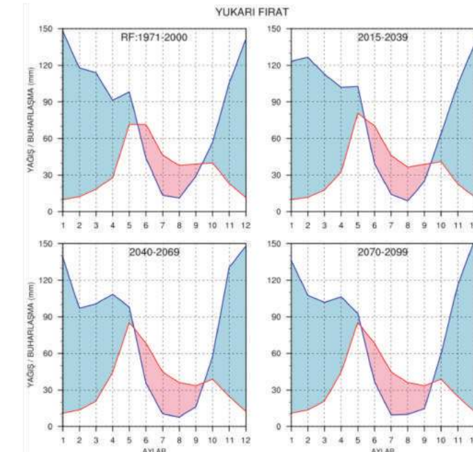
Şekil IV.27. Havza ortalaması alınmış Yukarı Fırat Tarım Havzası için RCP8.5 senaryosuna göre hesaplanmış olan, ortalama aylık toplam yağışın (mavi çizgi) ve gerçekleşen buharlaşma-terlemenin (kırmızı çizgi) yıl içindeki değişimine ait mevcut durum 1971-2000 ile birlikte bu mevcut duruma göre 2015-39, 2040-69 ve 2070-99 dönemleri için küresel iklim değişimi ile oluşan eğilim projeksiyonları.
