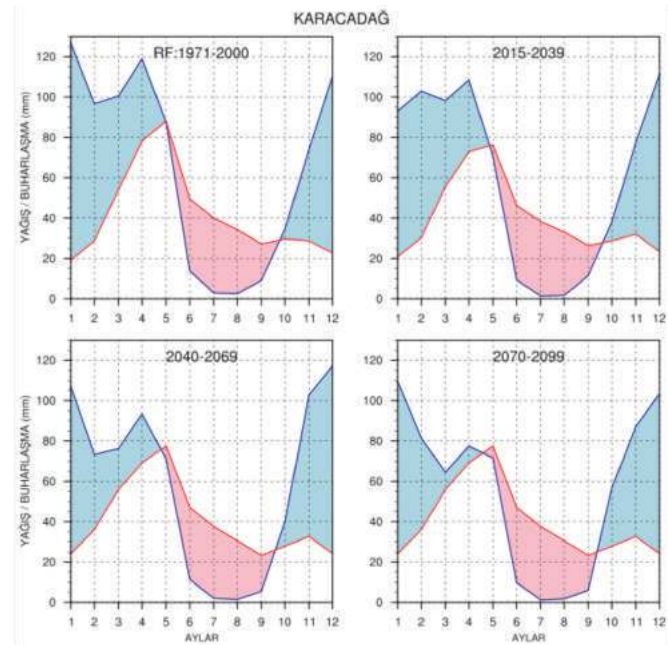
Şekil IV.14. Havza ortalaması alınmış Karacadağ Tarım Havzası için RCP8.5 senaryosuna göre hesaplanmış olan, ortalama aylık toplam yağışın (mavi çizgi) ve gerçekleşen buharlaşma-terlemenin (kırmızı çizgi) yıl içindeki değişimine ait mevcut durum 1971-2000 ile birlikte bu mevcut duruma göre 2015-39, 2040-69 ve 2070-99 dönemleri için küresel iklim değişimi ile oluşan eğilim projeksiyonları.
