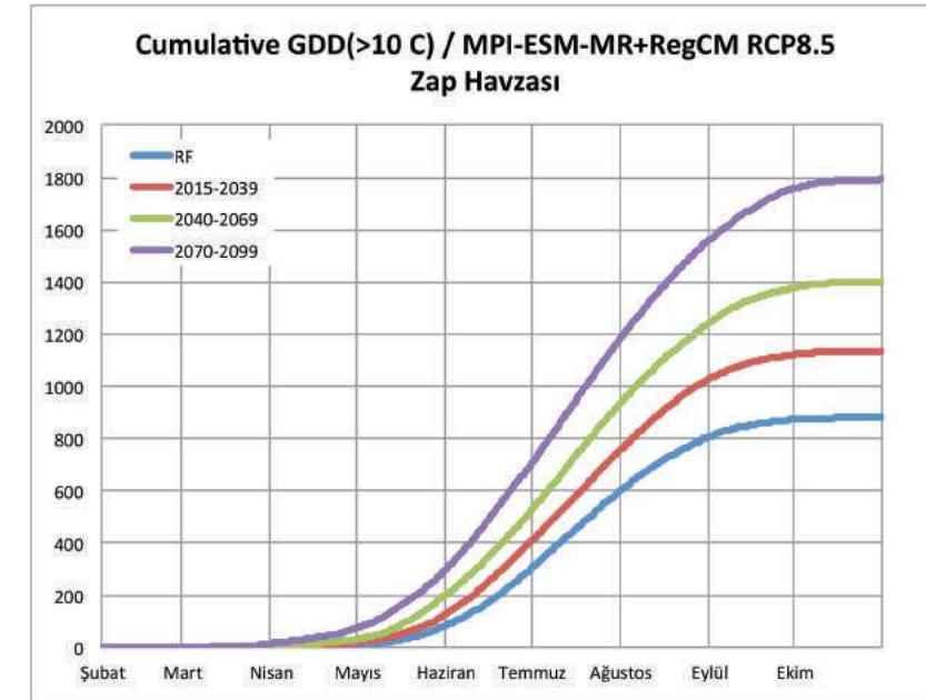
Şekil III.21. Havza ortalaması alınmış Zap Tarım Havzası için RCP8.5 senaryosuna göre hesaplanmış olan, ortalama günlük toprak sıcaklığı 10°C ve üzeri büyüme derece günlerinin yıl içindeki eklenik toplamına ait mevcut durum 1971-2000 (mavi çizgi) ile birlikte bu mevcut duruma göre 2015-39 (kırmızı çizgi), 2040-69 (yeşil çizgi) ve 2070-99 (mor çizgi) dönemleri için küresel iklim değişimi ile oluşan eğilim projeksiyonları.
