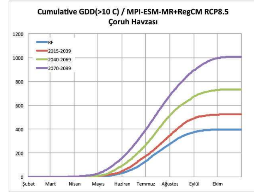
Şekil III.9. Havza ortalaması alınmış Çoruh Tarım Havzası için RCP8.5 senaryosuna göre hesaplanmış olan, ortalama günlük toprak sıcaklığı 10°C ve üzeri büyüme derece günlerinin yıl içindeki eklenik toplamlarına ait mevcut durum 1971-2000 (mavi çizgi) ile birlikte bu mevcut duruma göre 2015-39 (kırmızı çizgi), 2040-69 (yeşil çizgi) ve 2070-99 (mor çizgi) dönemleri için küresel iklim değişimi ile oluşan eğilim projeksiyonları.
