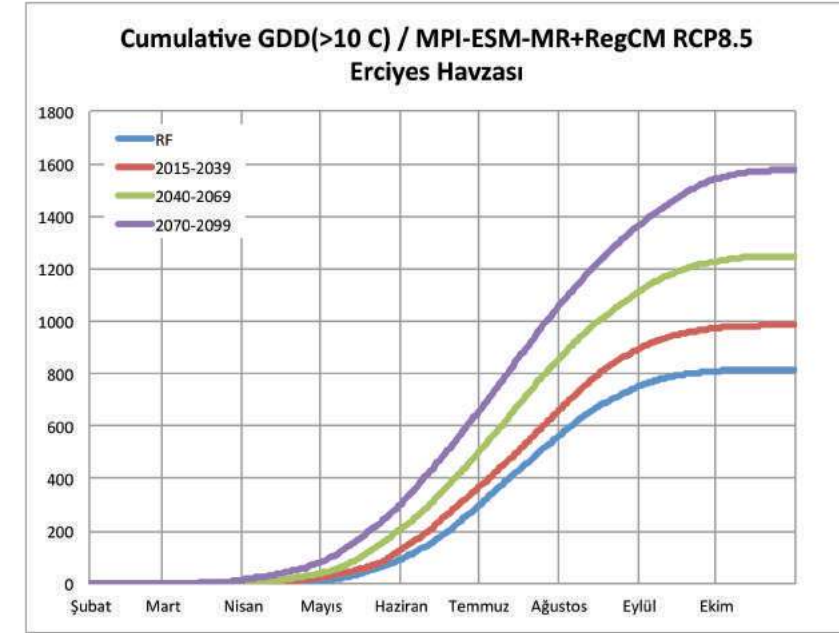
Şekil III.13. Havza ortalaması alınmış Erciyes Tarım Havzası için RCP8.5 senaryosuna göre hesaplanmış olan, ortalama günlük toprak sıcaklığı 10°C ve üzeri büyüme derece günlerinin yıl içindeki eklenik toplamına ait mevcut durum 1971-2000 (mavi çizgi) ile birlikte bu mevcut duruma göre 2015-39 (kırmızı çizgi), 2040-69 (yeşil çizgi) ve 2070-99 (mor çizgi) dönemleri için küresel iklim değişimi ile oluşan eğilim projeksiyonları.
