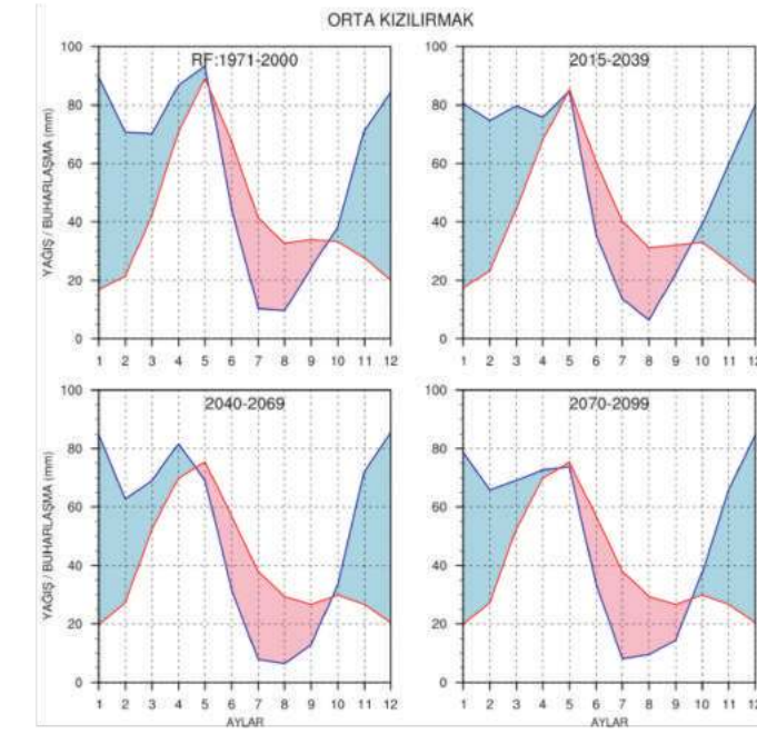
Şekil IV.23. Havza ortalaması alınmış Orta Kızılırmak Tarım Havzası için RCP8.5 senaryosuna göre hesaplanmış olan, ortalama aylık toplam yağışın (mavi çizgi) ve gerçekleşen buharlaşma-terlemenin (kırmızı çizgi) yıl içindeki değişimine ait mevcut durum 1971-2000 ile birlikte bu mevcut duruma göre 2015-39, 2040-69 ve 2070-99 dönemleri için küresel iklim değişimi ile oluşan eğilim projeksiyonları.
