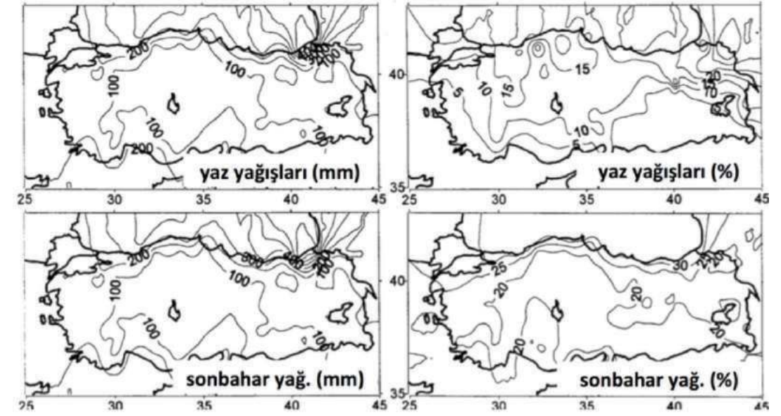
Şekil 3.3.4. Yaz ve sonbahar mevsimlerinde Türkiye üzerinde yağışların mevsimsel toplamı (mm) ve mevsim boyunca Türkiye genelinde alınan yıllık yağışa % olarak oranı, 1931-1990 (Kadioğlu, 2000).
