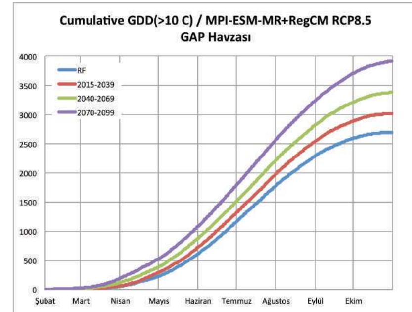
Şekil III.22. Havza ortalaması alınmış GAP Tarım Havzası için RCP8.5 senaryosuna göre hesaplanmış olan, ortalama günlük toprak sıcaklığı 10°C ve üzeri büyüme derece günlerinin yıl içindeki eklenik toplamına ait mevcut durum 1971-2000 (mavi çizgi) ile birlikte bu mevcut duruma göre 2015-39 (kırmızı çizgi), 2040-69 (yeşil çizgi) ve 2070-99 (mor çizgi) dönemleri için küresel iklim değişimi ile oluşan eğilim projeksiyonları.
