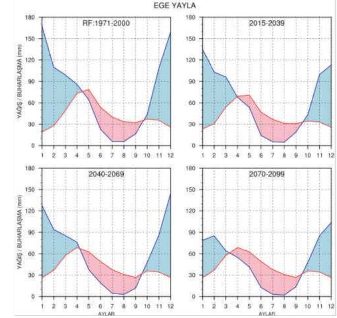
Şekil IV.7. Havza ortalaması alınmış Ege Yayla Tarım Havzası için RCP8.5 senaryosuna göre hesaplanmış olan, ortalama aylık toplam yağışın (mavi çizgi) ve gerçekleşen buharlaşma-terlemenin (kırmızı çizgi) yıl içindeki değişimine ait mevcut durum 1971-2000 ile birlikte bu mevcut duruma göre 2015-39, 2040-69 ve 2070-99 dönemleri için küresel iklim değişimi ile oluşan eğilim projeksiyonları.
