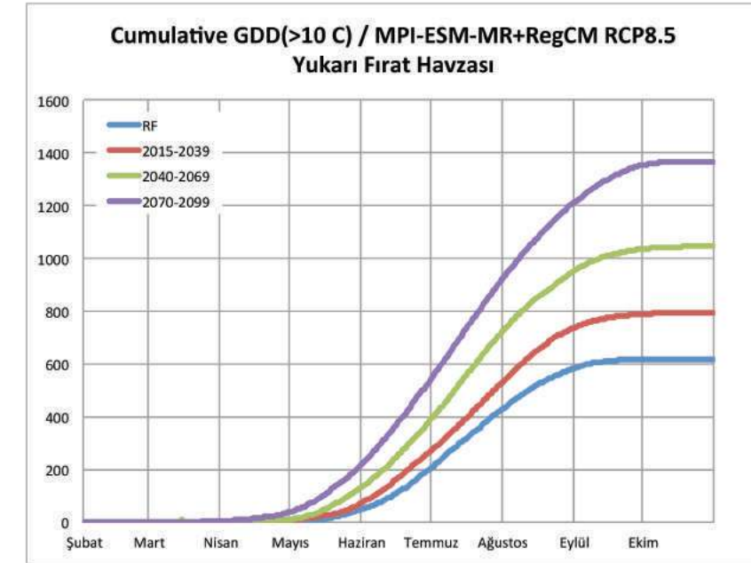
Şekil III.10. Havza ortalaması alınmış Yukarı Fırat Tarım Havzası için RCP8.5 senaryosuna göre hesaplanmış olan, ortalama günlük toprak sıcaklığı 10°C ve üzeri büyüme derece günlerinin yıl içindeki eklenik toplamlarına ait mevcut durum 1971-2000 (mavi çizgi) ile birlikte bu mevcut duruma göre 2015-39 (kırmızı çizgi), 2040-69 (yeşil çizgi) ve 2070-99 (mor çizgi) dönemleri için küresel iklim değişimi ile oluşan eğilim projeksiyonları.
