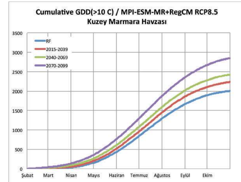
Şekil III.6. Havza ortalaması alınmış Kuzey Marmara Tarım Havzası için RCP8.5 senaryosuna göre hesaplanmış olan, ortalama günlük toprak sıcaklığı 10°C ve üzeri büyüme derece günlerinin yıl içindeki eklenik toplamına ait mevcut durum 1971-2000 (mavi çizgi) ile birlikte bu mevcut duruma göre 2015-39 (kırmızı çizgi), 2040-69 (yeşil çizgi) ve 2070-99 (mor çizgi) dönemleri için küresel iklim değişimi ile oluşan eğilim projeksiyonları.
