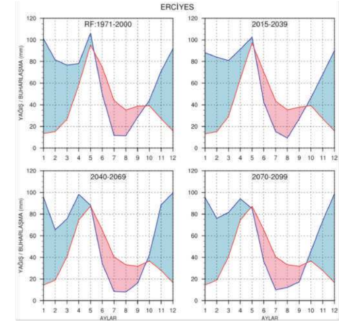
Şekil IV.8. Havza ortalaması alınmış Erciyes Tarım Havzası için RCP8.5 senaryosuna göre hesaplanmış olan, ortalama aylık toplam yağışın (mavi çizgi) ve gerçekleşen buharlaşma-terlemenin (kırmızı çizgi) yıl içindeki değişimine ait mevcut durum 1971-2000 ile birlikte bu mevcut duruma göre 2015-39, 2040-69 ve 2070-99 dönemleri için küresel iklim değişimi ile oluşan eğilim projeksiyonları.
