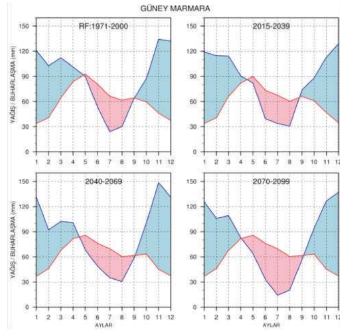
Şekil IV.13. Havza ortalaması alınmış Güney Marmara Tarım Havzası için RCP8.5 senaryosuna göre hesaplanmış olan, ortalama aylık toplam yağışın (mavi çizgi) ve gerçekleşen buharlaşma-terlemenin (kırmızı çizgi) yıl içindeki değişimine ait mevcut durum 1971-2000 ile birlikte bu mevcut duruma göre 2015-39, 2040-69 ve 2070-99 dönemleri için küresel iklim değişimi ile oluşan eğilim projeksiyonları.
