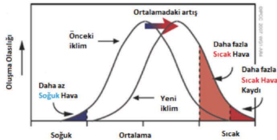
Şekil 3.5.11. Normal sıcaklık dağılımında ortalama hava sıcaklığındaki değişimi aşırı değerleri nasıl değiştireceğinin şematik gösterimi (IPCC, 2007).
