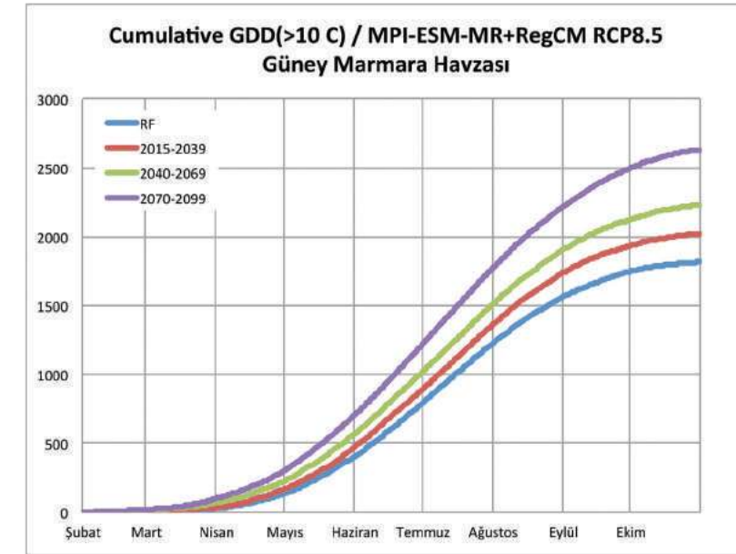
Şekil III.1. Havza ortalaması alınmış Güney Marmara Tarım Havzası için RCP8.5 senaryosuna göre hesaplanmış olan, ortalama günlük toprak sıcaklığı 10°C ve üzeri büyüme derece günlerinin yıl içindeki eklenik toplamına ait mevcut durum 1971-2000 (mavi çizgi) ile birlikte bu mevcut duruma göre 2015-39 (kırmızı çizgi), 2040-69 (yeşil çizgi) ve 2070-99 (mor çizgi) dönemleri için küresel iklim değişikliği ile oluşan eğilim projeksiyonları.
