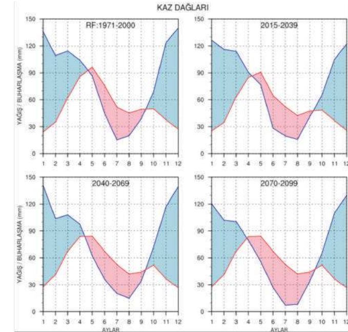
Şekil IV.16. Havza ortalaması alınmış Kaz Dağları Tarım Havzası için RCP8.5 senaryosuna göre hesaplanmış olan, ortalama aylık toplam yağışın (mavi çizgi) ve gerçekleşen buharlaşma-terlemenin (kırmızı çizgi) yıl içindeki değişimine ait mevcut durum 1971-2000 ile birlikte bu mevcut duruma göre 2015-39, 2040-69 ve 2070-99 dönemleri için küresel iklim değişimi ile oluşan eğilim projeksiyonları.
