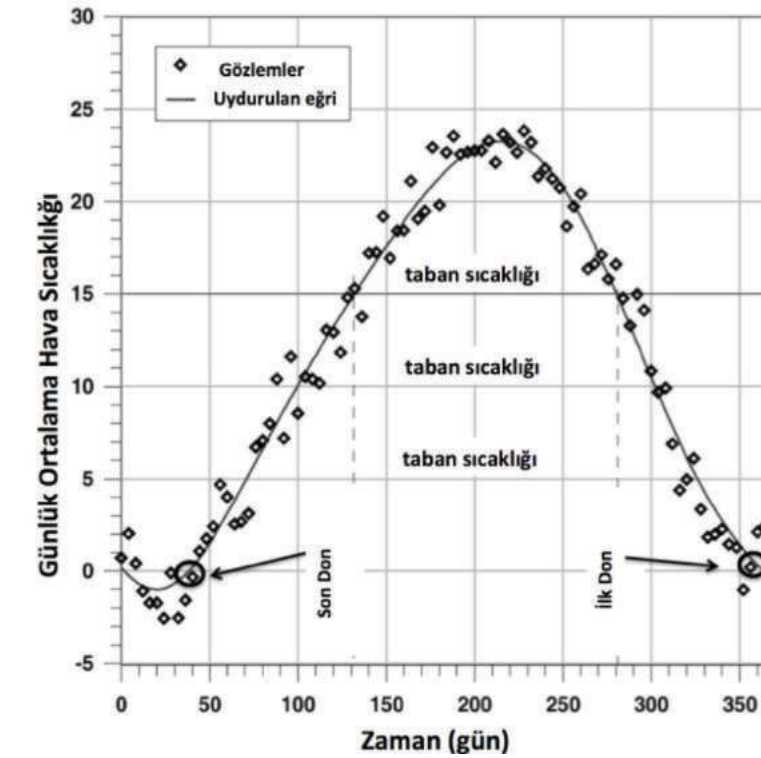
Şekil 3.2.1. Yıl içindeki günlük ortalama hava sıcaklıklarının değişimi ile birlikte büyüme mevsimini gösteren son ve ilk don tarihlerinin olası taban sıcaklıklarının şematik gösterimi.
