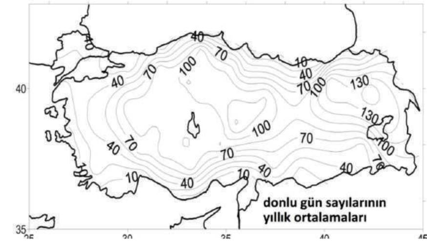
Şekil 3.2.3. 1961-1990 yılları ortalamasına göre Türkiye genelinde görülen donlu gün sayılarının yıllık ortalamaları
