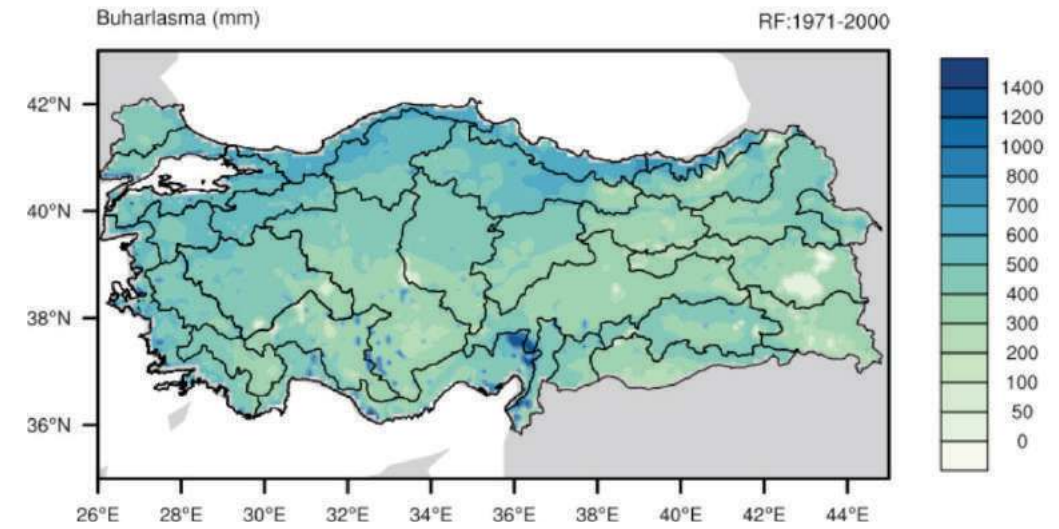
Şekil 3.3.8. MPI-ESM-MR+RegCM Modeli RCP8.5 Senaryosuna göre 1971-2000 referans dönemi bitki büyüme mevsiminde (Mart-Ekim) beklenen toplam gerçek buharlaşma-terleme miktarları.
