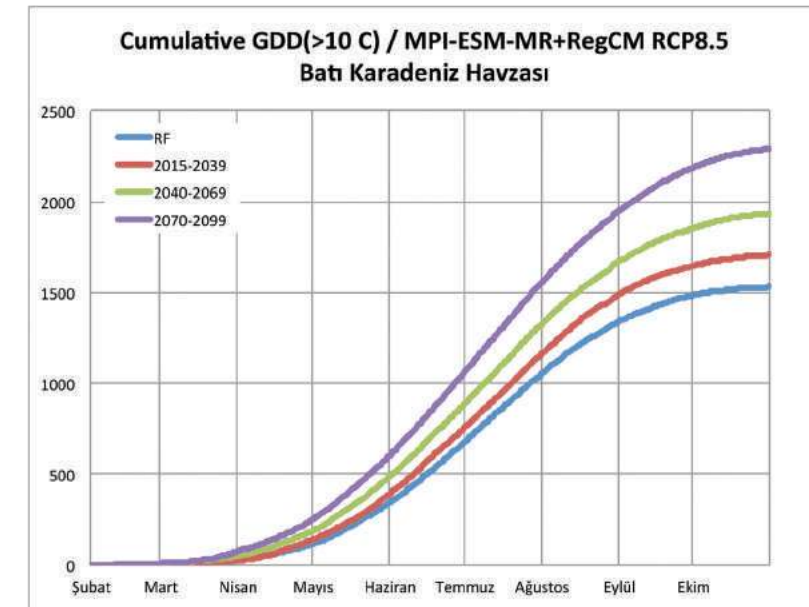
Şekil III.2. Havza ortalaması alınmış Batı Karadeniz Tarım Havzası için RCP8.5 senaryosuna göre hesaplanmış olan, ortalama günlük toprak sıcaklığı 10°C ve üzeri büyüme derece günlerinin yıl içindeki eklenik toplamına ait mevcut durum 1971-2000 (mavi çizgi) ile birlikte bu mevcut duruma göre 2015-39 (kırmızı çizgi), 2040-69 (yeşil çizgi) ve 2070-99 (mor çizgi) dönemleri için küresel iklim değişikliği ile oluşan eğilim projeksiyonları.
