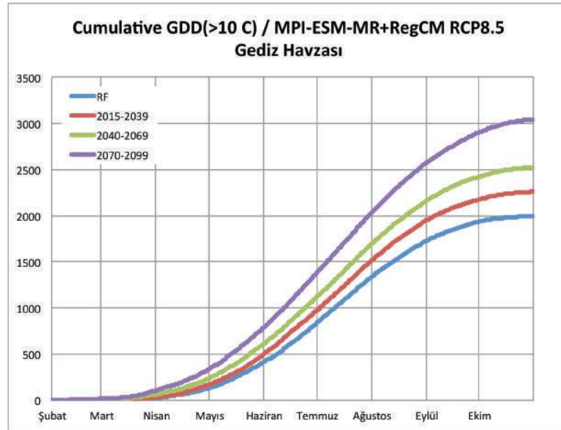
Şekil III.16. Havza ortalaması alınmış Gediz Tarım Havzası için RCP8.5 senaryosuna göre hesaplanmış olan, ortalama günlük toprak sıcaklığı 10°C ve üzeri büyüme derece günlerinin yıl içindeki eklenik toplamalarına ait mevcut durum 1971-2000 (mavi çizgi) ile birlikte bu mevcut duruma göre 2015-39 (kırmızı çizgi), 2040-69 (yeşil çizgi) ve 2070-99 (mor çizgi) dönemleri için küresel iklim değişimi ile oluşan eğilim projeksiyonları.
