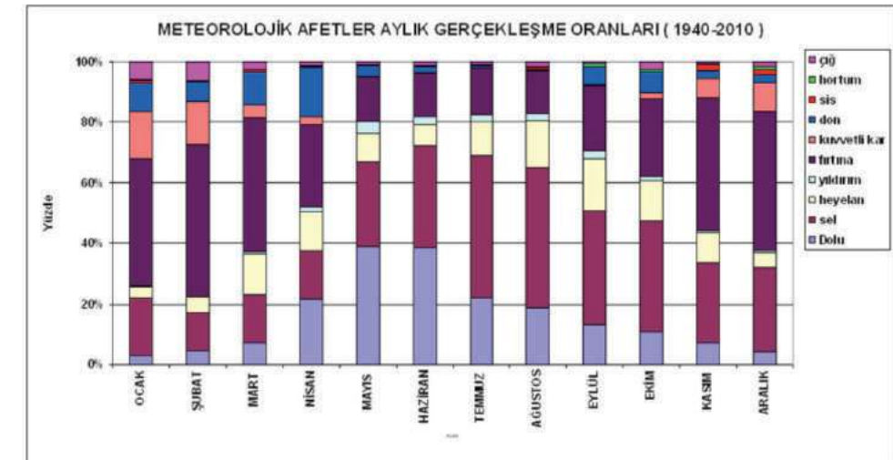
Şekil 3.5.10. Türkiye’de hidro-meteorolojik afet oluşumlarının aylara göre dağılımı.
