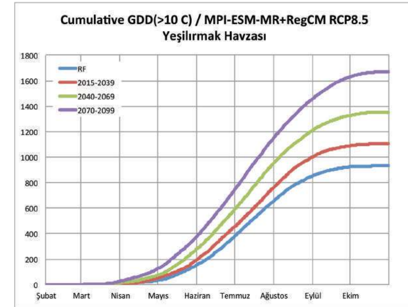
Şekil III.18. Havza ortalaması alınmış Yeşilirmak Tarım Havzası için RCP8.5 senaryosuna göre hesaplanmış olan, ortalama günlük toprak sıcaklığı 10°C ve üzeri büyüme derece günlerinin yıl içindeki eklenik toplamalarına ait mevcut durum 1971-2000 (mavi çizgi) ile birlikte bu mevcut duruma göre 2015-39 (kırmızı çizgi), 2040-69 (yeşil çizgi) ve 2070-99 (mor çizgi) dönemleri için küresel iklim değişimi ile oluşan eğilim projeksiyonları.
