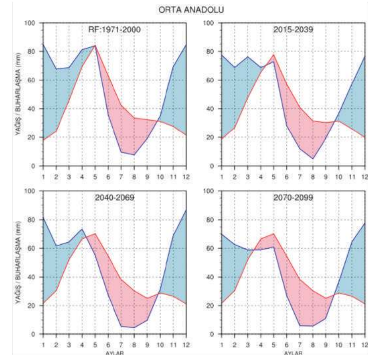
Şekil 3.4.2. Havza ortalaması alınmış Orta Anadolu Tarım Havzası için RCP8.5 senaryosuna göre hesaplanmış olan, ortalama aylık toplam yağışın (mavi çizgi) ve gerçekleşen buharlaşma-terlemenin (kırmızı çizgi) yıl içindeki değişimine ait mevcut durum 1971-2000 ile birlikte bu mevcut duruma göre 2015-2039, 2040-2069 ve 2070-2099 dönemleri için küresel iklim değişimi ile oluşan eğilim projeksiyonları.
