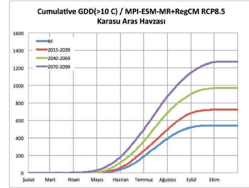
Şekil III.5. Havza ortalaması alınmış Karasu Aras Tarım Havzası için RCP8.5 senaryosuna göre hesaplanmış olan, ortalama günlük toprak sıcaklığı 10°C ve üzeri büyüme derece günlerinin yıl içindeki eklenik toplamına ait mevcut durum 1971-2000 (mavi çizgi) ile birlikte bu mevcut duruma göre 2015-39 (kırmızı çizgi), 2040-69 (yeşil çizgi) ve 2070-99 (mor çizgi) dönemleri için küresel iklim değişimi ile oluşan eğilim projeksiyonları.
