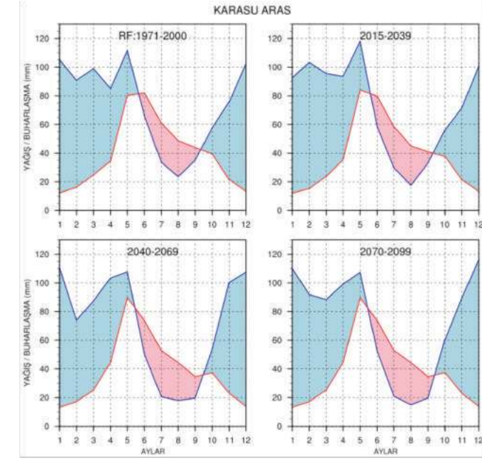
Şekil IV.15. Havza ortalaması alınmış Karasu Aras Tarım Havzası için RCP8.5 senaryosuna göre hesaplanmış olan, ortalama aylık toplam yağışın (mavi çizgi) ve gerçekleşen buharlaşma-terlemenin (kırmızı çizgi) yıl içindeki değişimine ait mevcut durum 1971-2000 ile birlikte bu mevcut duruma göre 2015-39, 2040-69 ve 2070-99 dönemleri için küresel iklim değişimi ile oluşan eğilim projeksiyonları.
