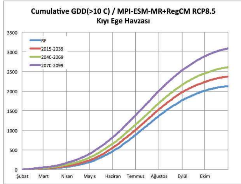
Şekil III.11. Havza ortalaması alınmış Kıy Ege Tarım Havzası için RCP8.5 senaryosuna göre hesaplanmış olan, ortalama günlük toprak sıcaklığı 10°C ve üzeri büyüme derece günlerinin yıl içindeki eklenik toplamına ait mevcut durum 1971-2000 (mavi çizgi) ile birlikte bu mevcut duruma göre 2015-39 (kırmızı çizgi), 2040-69 (yeşil çizgi) ve 2070-99 (mor çizgi) dönemleri için küresel iklim değişimi ile oluşan eğilim projeksiyonları.
