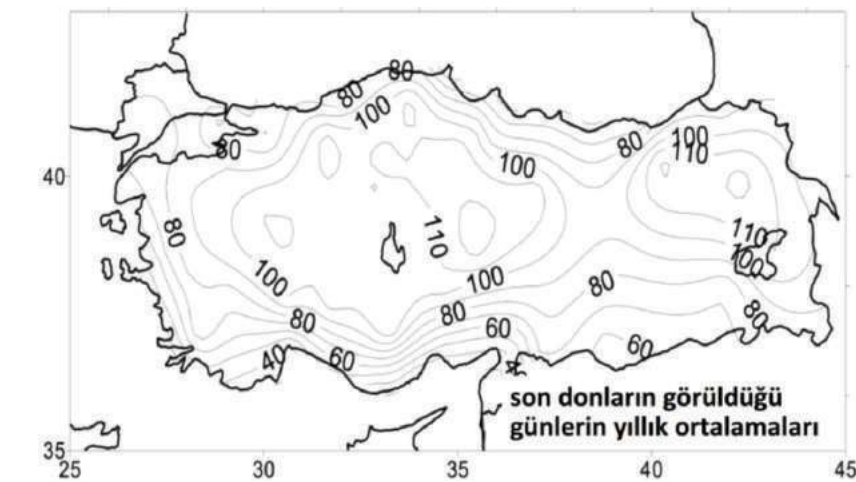
Şekil 3.2.4. 1961-1990 yılları ortalamasına göre genellikle ilkbaharda görülen son donların yıllık ortalaması.
