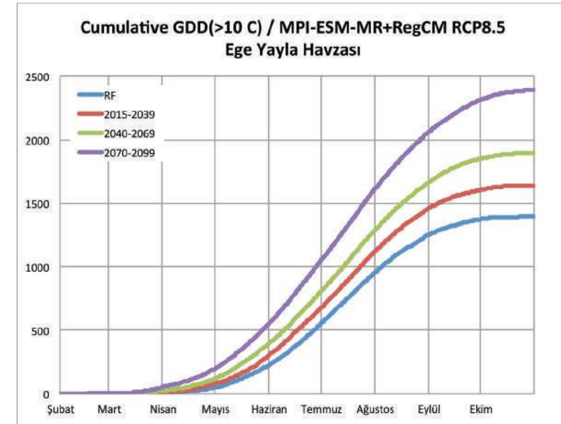
Şekil III.26. Havza ortalaması alınmış Ege Yayla Tarım Havzası için RCP8.5 senaryosuna göre hesaplanmış olan, ortalama günlük toprak sıcaklığı 10°C ve üzeri büyüme derece günlerinin yıl içindeki eklenik toplamlarına ait mevcut durum 1971-2000 (mavi çizgi) ile birlikte bu mevcut duruma göre 2015-39 (kırmızı çizgi), 2040-69 (yeşil çizgi) ve 2070-99 (mor çizgi) dönemleri için küresel iklim değişimi ile oluşan eğilim projeksiyonları.
