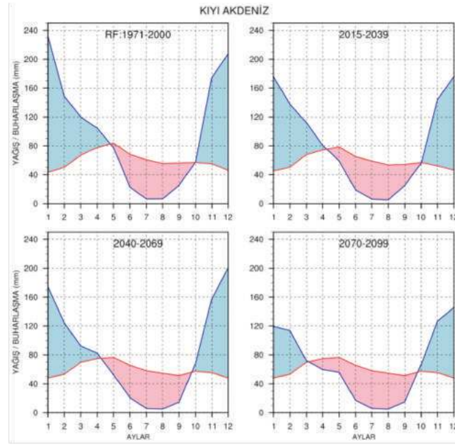
Şekil IV.17. Havza ortalaması alınmış Kiyi Akdeniz Tarım Havzası için RCP8.5 senaryosuna göre hesaplanmış olan, ortalama aylık toplam yağışın (mavi çizgi) ve gerçekleşen buharlaşma-terlemenin (kırmızı çizgi) yıl içindeki değişimine ait mevcut durum 1971-2000 ile birlikte bu mevcut duruma göre 2015-39, 2040-69 ve 2070-99 dönemleri için küresel iklim değişimi ile oluşan eğilim projeksiyonları.
