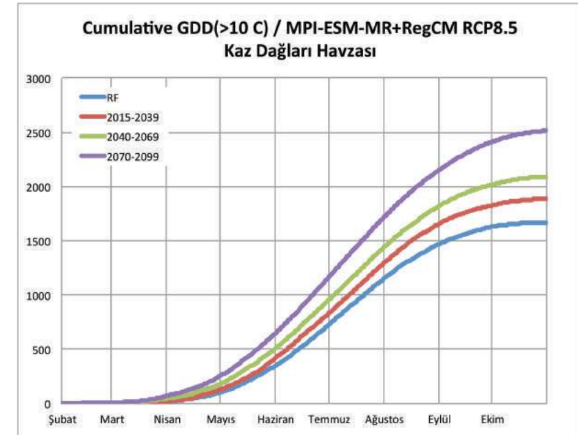
Şekil III.14. Havza ortalaması alınmış Kaz Dağları Tarım Havzası için RCP8.5 senaryosuna göre hesaplanmış olan, ortalama günlük toprak sıcaklığı 10°C ve üzeri büyüme derece günlerinin yıl içindeki eklenik toplamına ait mevcut durum 1971-2000 (mavi çizgi) ile birlikte bu mevcut duruma göre 2015-39 (kırmızı çizgi), 2040-69 (yeşil çizgi) ve 2070-99 (mor çizgi) dönemleri için küresel iklim değişimi ile oluşan eğilim projeksiyonları.
