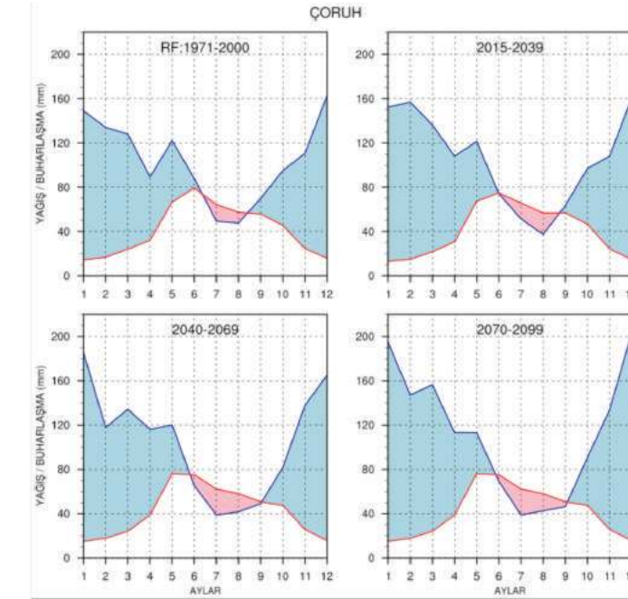
Şekil IV.4. Havza ortalaması alınmış Çoruh Tarım Havzası için RCP8.5 senaryosuna göre hesaplanmış olan, ortalama aylık toplam yağışın (mavi çizgi) ve gerçekleşen buharlaşma-terlemenin (kırmızı çizgi) yıl içindeki değişimine ait mevcut durum 1971-2000 ile birlikte bu mevcut duruma göre 2015-39, 2040-69 ve 2070-99 dönemleri için küresel iklim değişikliği ile oluşan eğilim projeksiyonları.
