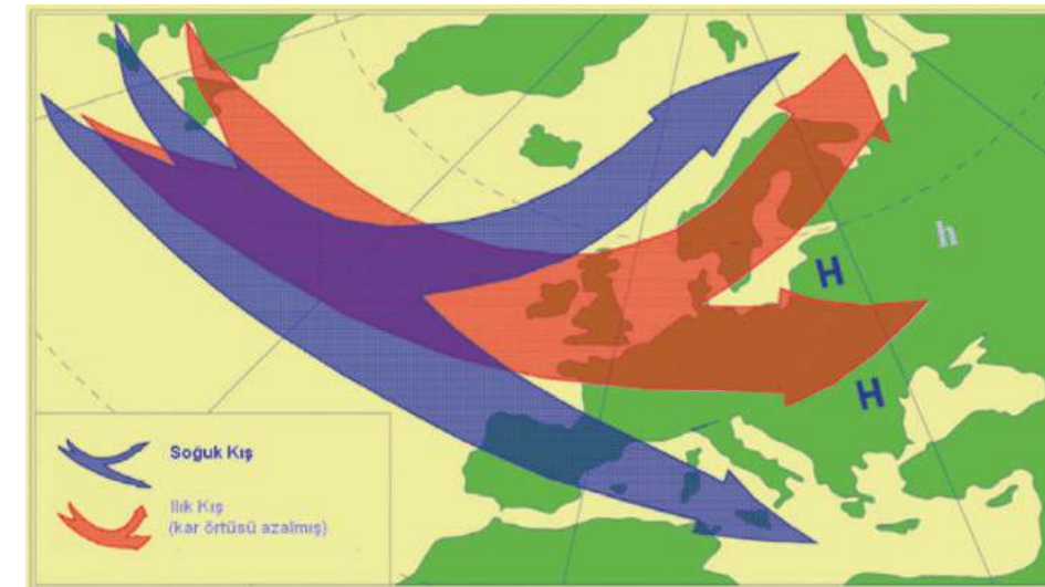
Şekil 3.3. Yüksek basınç merkezlerinin engellemesi ile birlikte soğuk ve sıcak Avrupa kışlarında fırtına yörüngeleri (Dronia, 1991).
