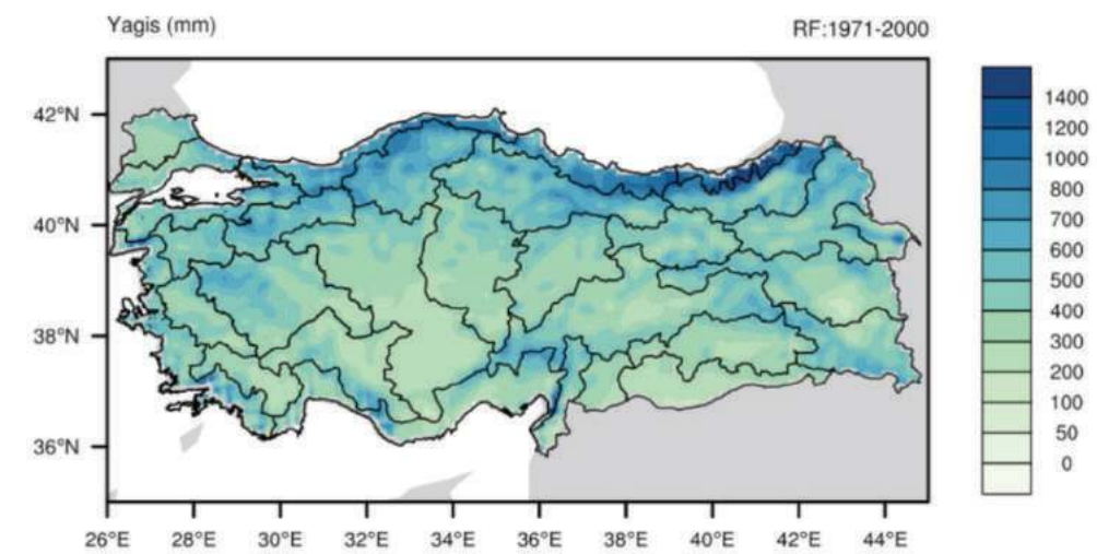
Şekil 3.3.6. MPI-ESM-MR+RegCM Modeli RCP8.5 Senaryosuna göre 1971-2000 referans dönemi bitki büyüme mevsimindeki (Mart-Ekim) toplam yağış.
