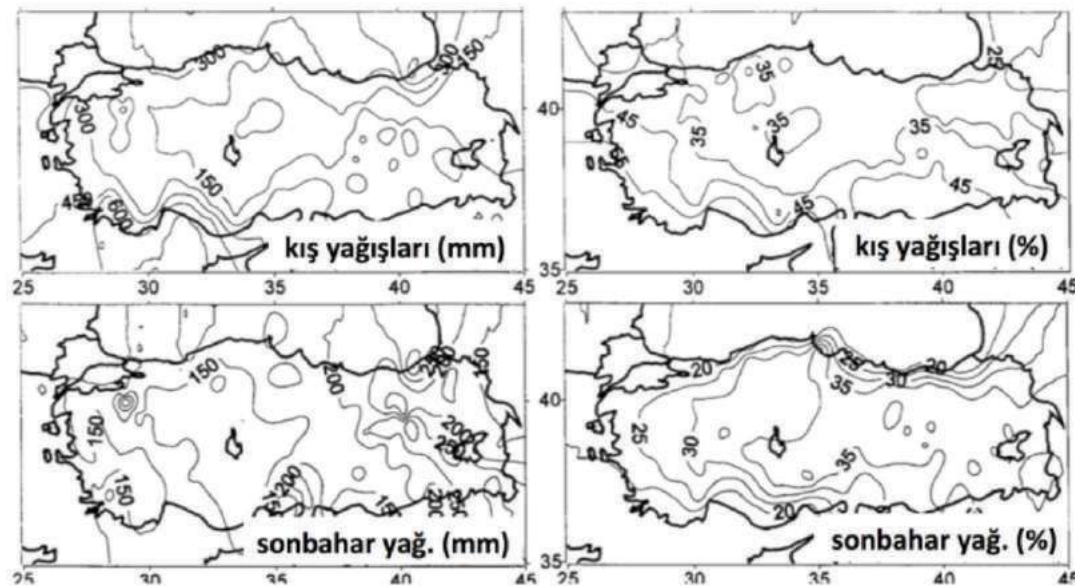
Şekil 3.3.3. Kış ve sonbahar mevsimlerinde Türkiye üzerinde yağışların mevsimsel toplamı (mm) ve mevsim boyunca Türkiye genelinde alınan yıllık yağışa % olarak oranı, 1931-1990 (Kadioğlu, 2000).
