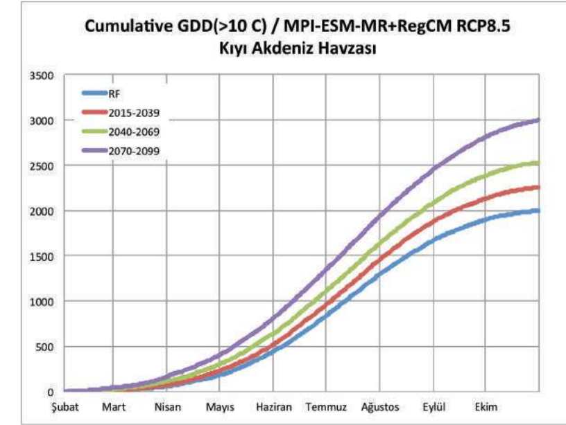
Şekil III.25. Havza ortalaması alınmış Kıyı Akdeniz Tarım Havzası için RCP8.5 senaryosuna göre hesaplanmış olan, ortalama günlük toprak sıcaklığı 10°C ve üzeri büyüme derece günlerinin yıl içindeki eklenik toplamlarına ait mevcut durum 1971-2000 (mavi çizgi) ile birlikte bu mevcut duruma göre 2015-39 (kırmızı çizgi), 2040-69 (yeşil çizgi) ve 2070-99 (mor çizgi) dönemleri için küresel iklim değişimi ile oluşan eğilim projeksiyonları.
