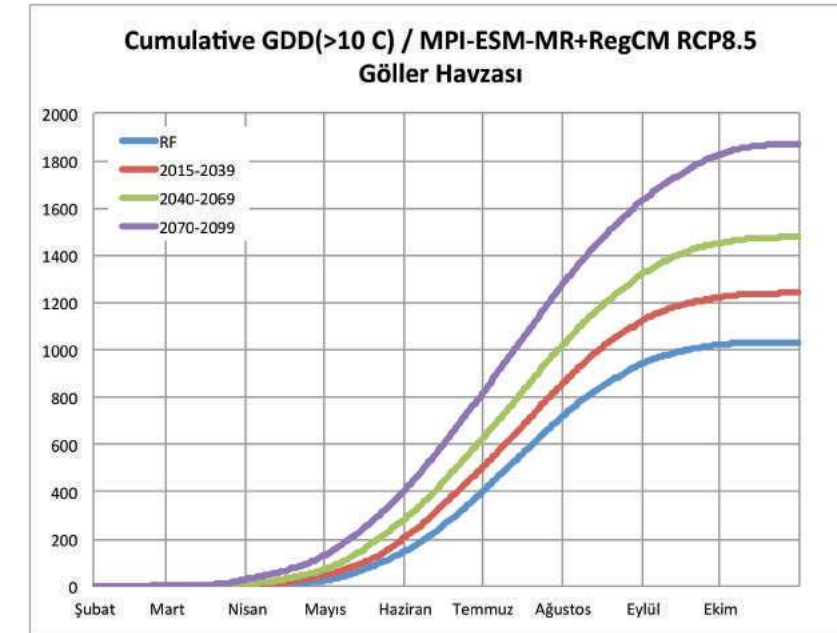
Şekil III.29. Havza ortalaması alınmış Göller Tarım Havzası için RCP8.5 senaryosuna göre hesaplanmış olan, ortalama günlük toprak sıcaklığı 10°C ve üzeri büyüme derece günlerinin yıl içindeki eklenik toplamına ait mevcut durum 1971-2000 (mavi çizgi) ile birlikte bu mevcut duruma göre 2015-39 (kırmızı çizgi), 2040-69 (yeşil çizgi) ve 2070-99 (mor çizgi) dönemleri için küresel iklim değişimi ile oluşan eğilim projeksiyonları.
