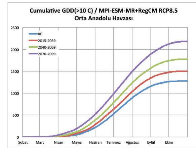
Şekil 3.2.9. Orta Anadolu Tarım Havzası için ortalama günlük toprak sıcaklığı 10°C ve üzeri büyüme derece günlerinin yıl içindeki eklenik toplamına ait mevcut durum 1971-2000 (mavi çizgi) ile birlikte RCP8.5 senaryosuna göre gelecek 2015-39 (kırmızı çizgi), 2040-2069 (yeşil çizgi) ve 2070-2099 (mor çizgi) dönemleri için küresel iklim değişimi ile oluşan eğilim projeksiyonları.
