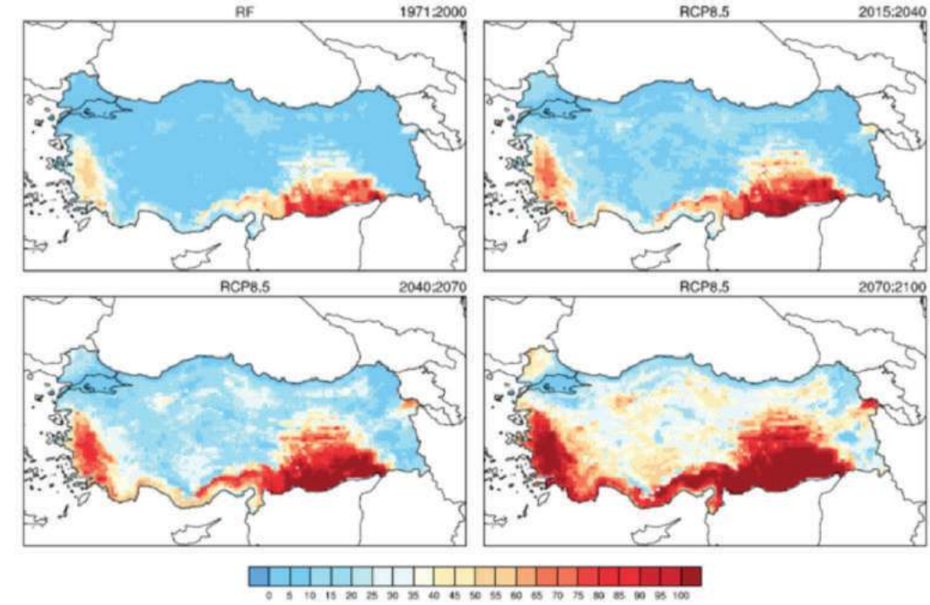
Şekil 3.5.12. MPI-ESM-MR Modeli RCP8.5 Senaryosuna göre 30 yıllık Çok Sıcak Gün (TX35) İklim İndisi değerlerinin belirtilen periyot içerisindeki yıllık ortalamaları (gün).
